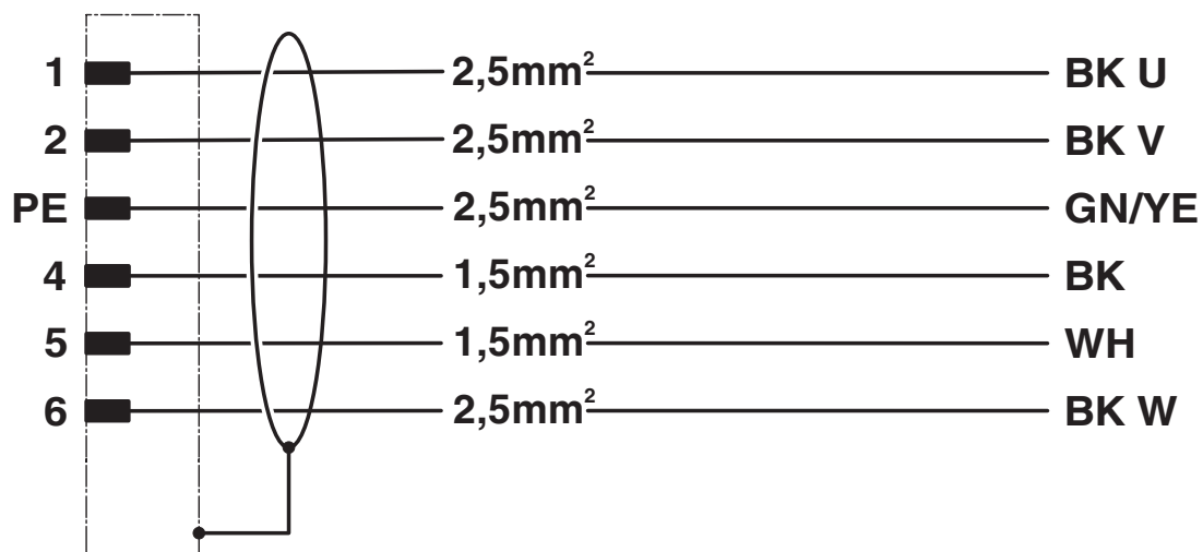
Schaltplan
