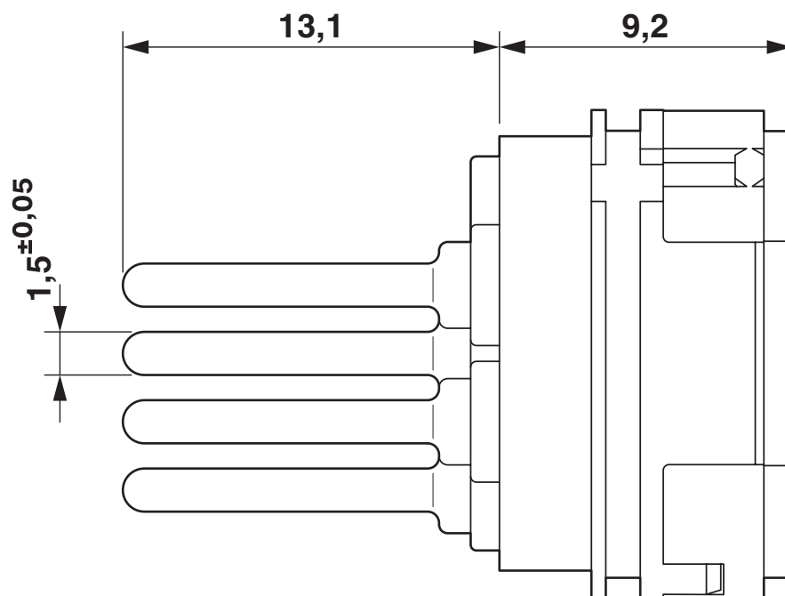
Maßzeichnung
