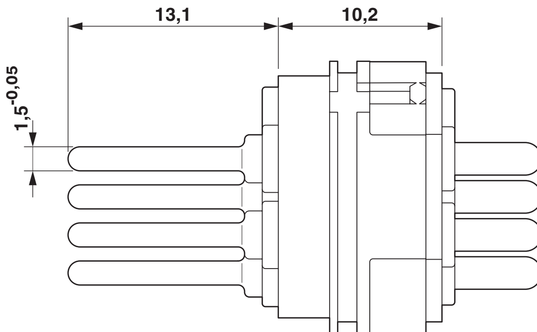
Maßzeichnung
