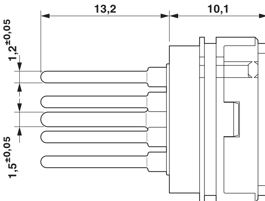
Maßzeichnung
