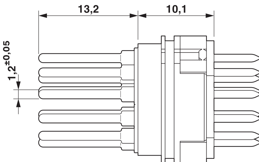
Maßzeichnung
