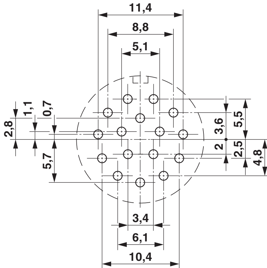
Bohrplan/Lötpadgeometrie
