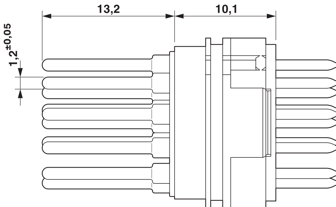
Maßzeichnung
