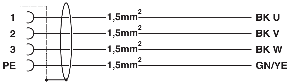
Schaltplan
