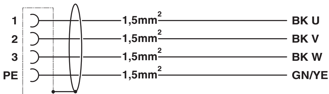
Schaltplan
