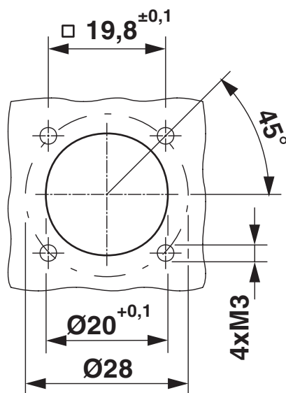
Schemazeichnung
