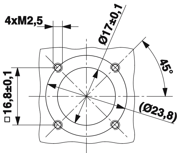
Maßzeichnung
