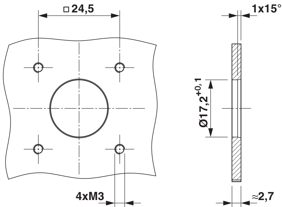
Maßzeichnung
