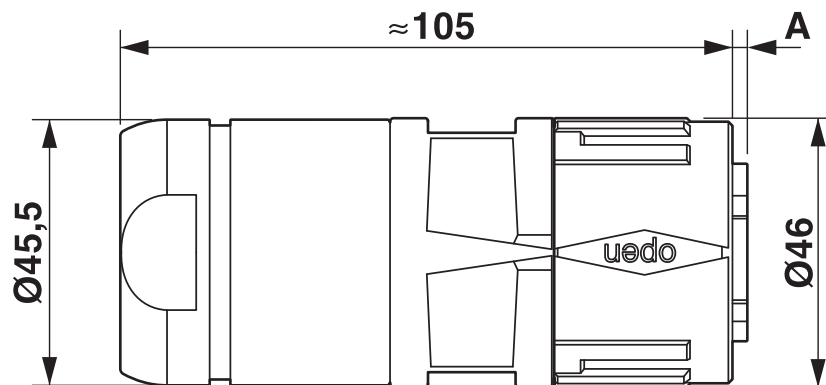
Maßzeichnung
