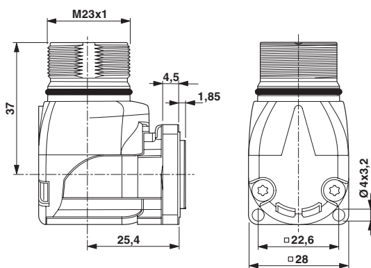
Maßzeichnung
