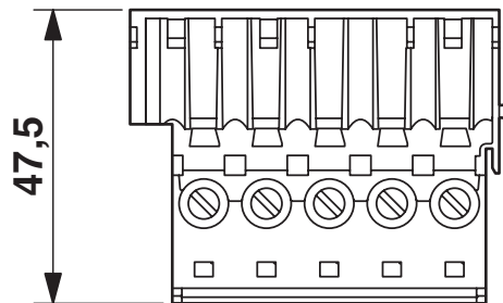
Maßzeichnung
