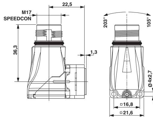
Maßzeichnung
