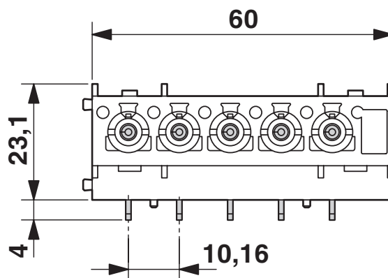
Maßzeichnung
