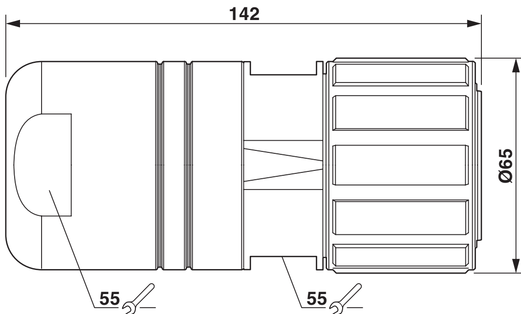
Maßzeichnung
