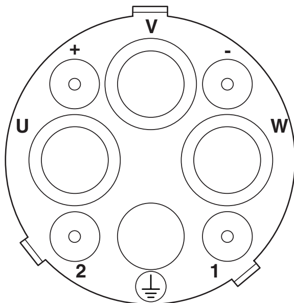
Schemazeichnung
