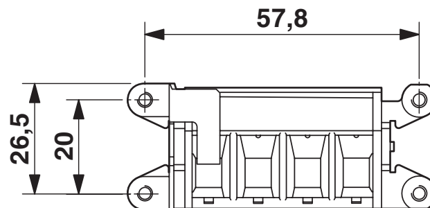
Maßzeichnung
