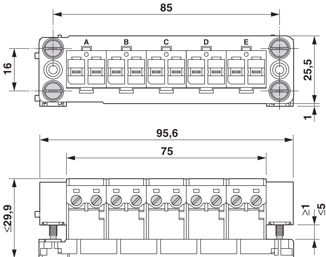
Maßzeichnung
