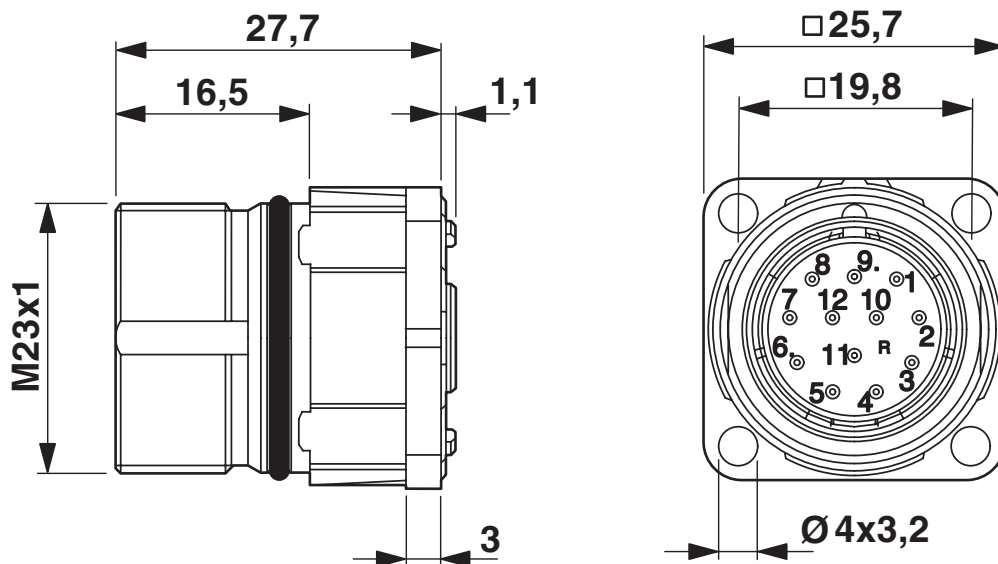
Maßzeichnung
