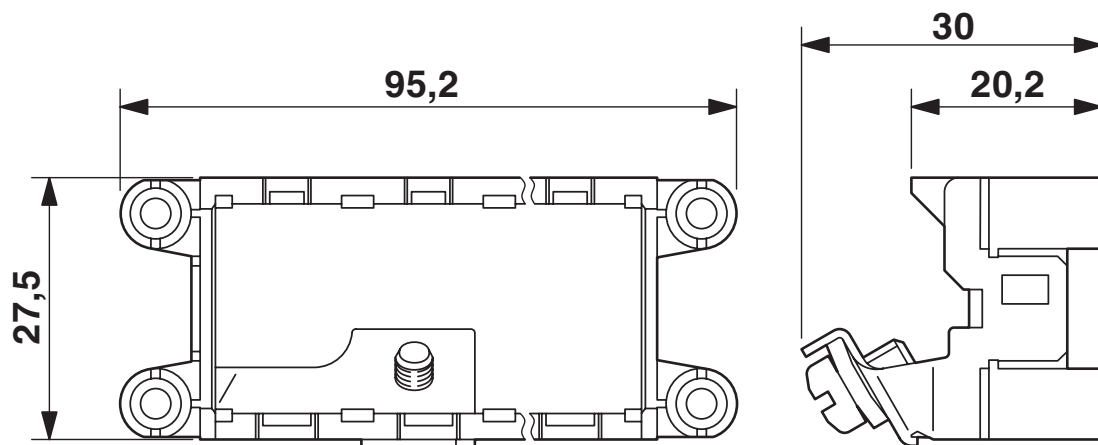
Maßzeichnung
