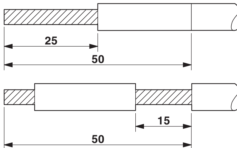
Funktionszeichnung
