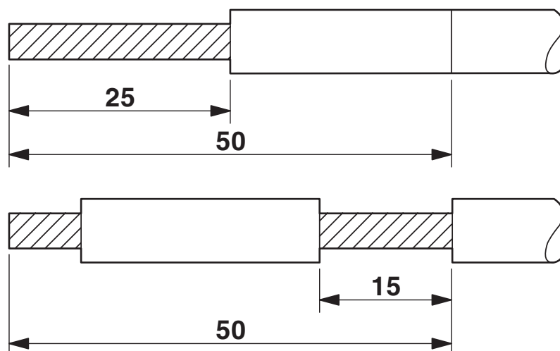
Funktionszeichnung
