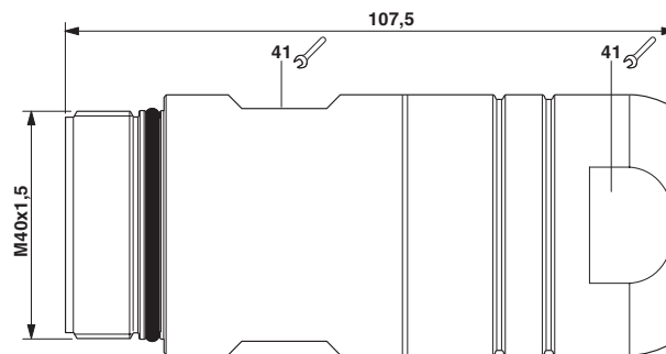
Maßzeichnung
