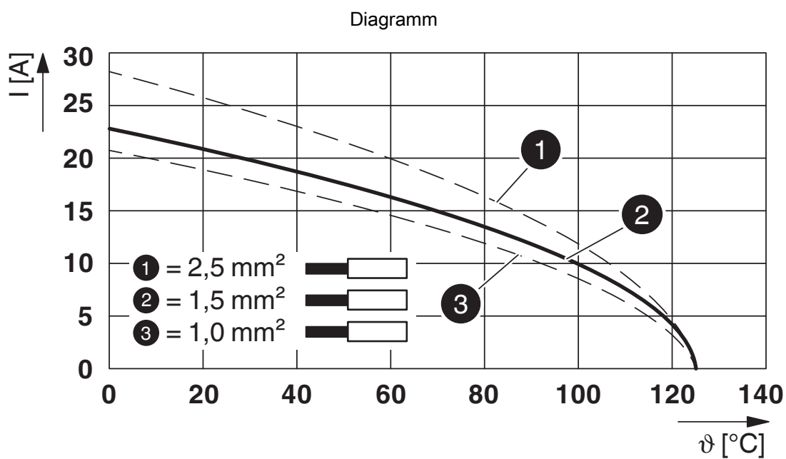
Derating-Diagramm für starre Leiter
