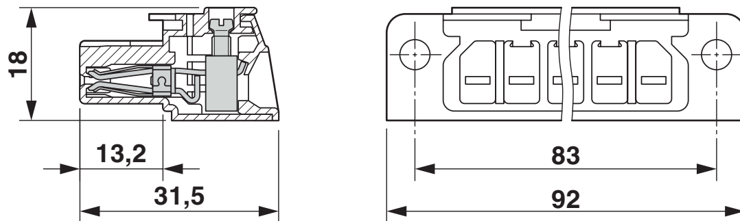
Maßzeichnung
