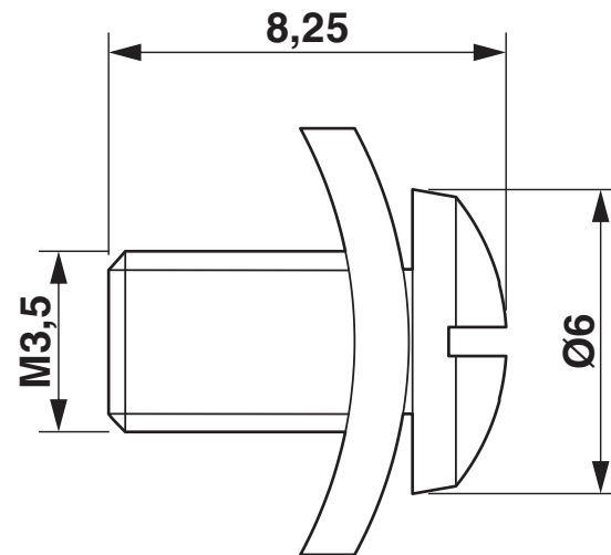
Maßzeichnung
