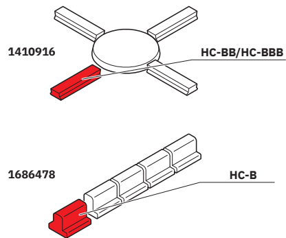
Schemazeichnung
