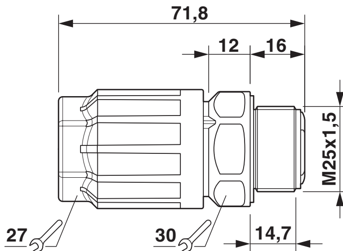
Maßzeichnung
