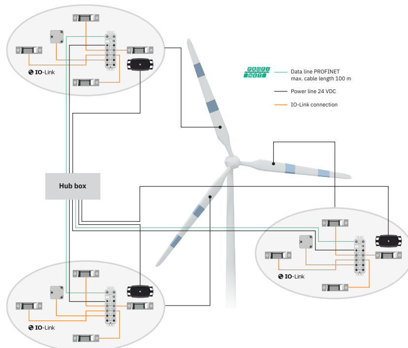
Applikationszeichnung
