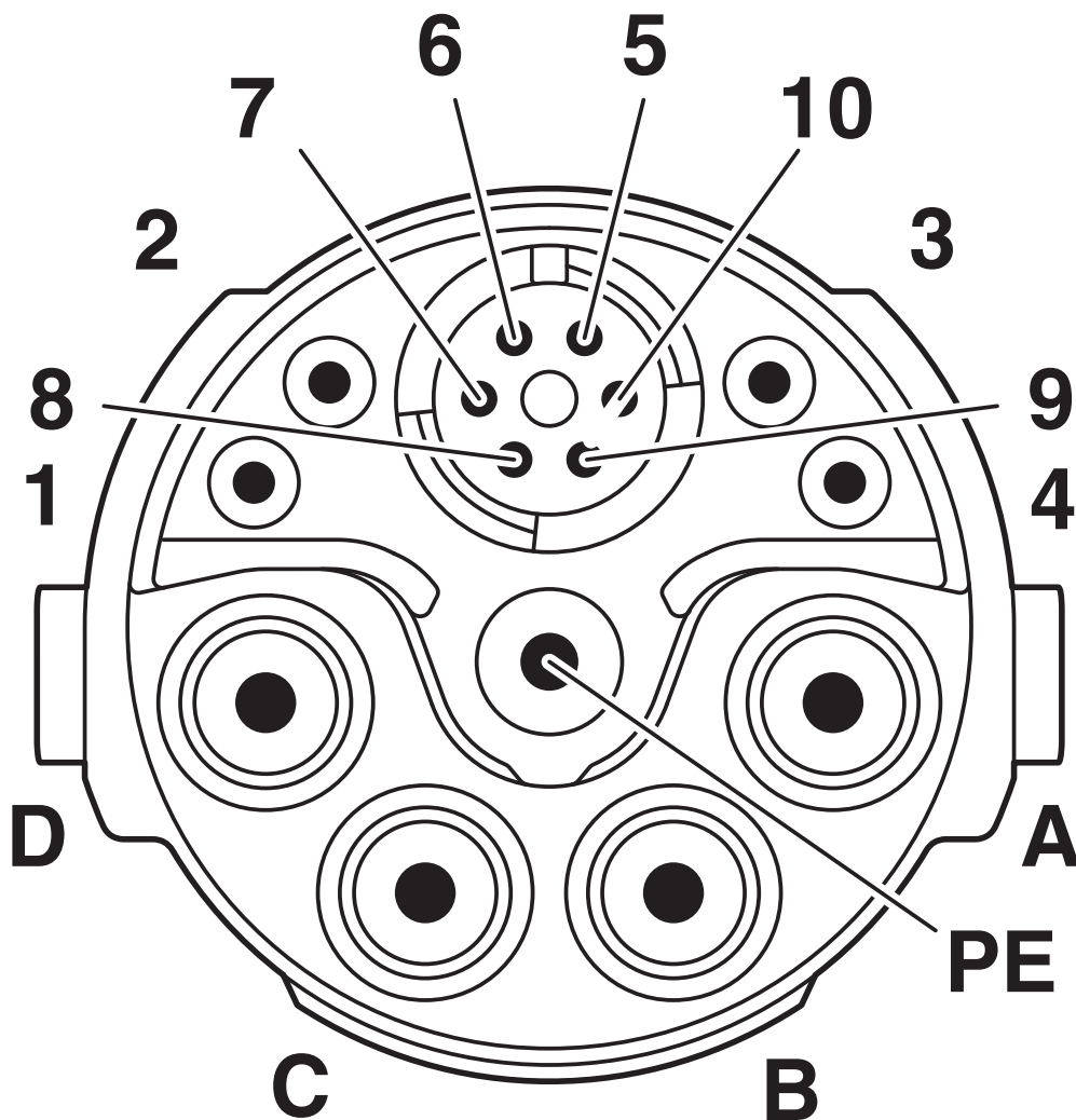
Schemazeichnung
