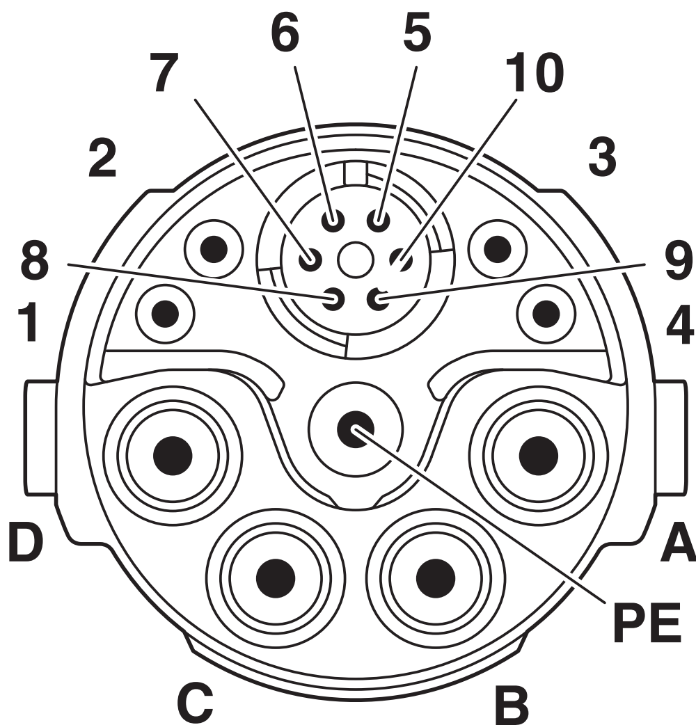
Schemazeichnung
