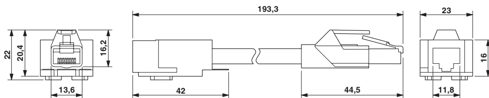
Maßzeichnung
