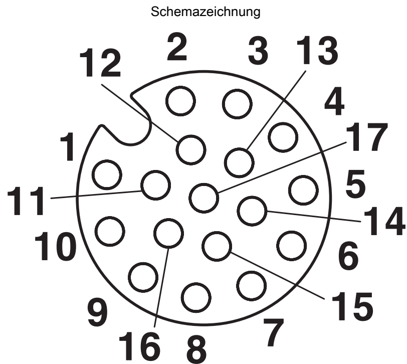
Polbild Buchse M12, 17-polig, Ansicht Buchsenseite
