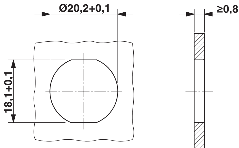
Maßzeichnung
