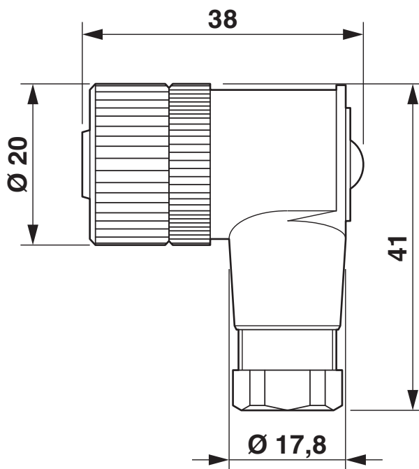
Maßzeichnung
