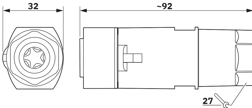
Maßzeichnung
