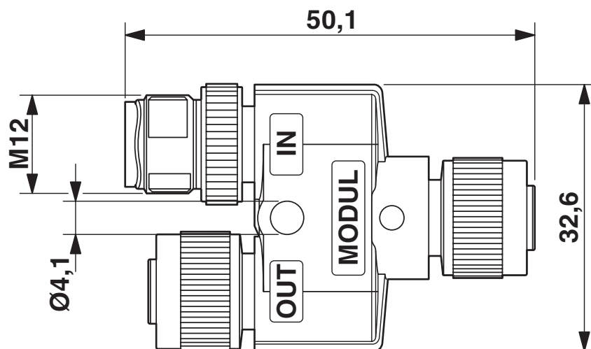
Maßzeichnung
