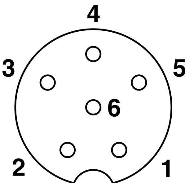
Schemazeichnung
