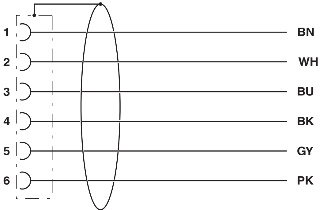
Kontaktbelegung der M8-Buchse
