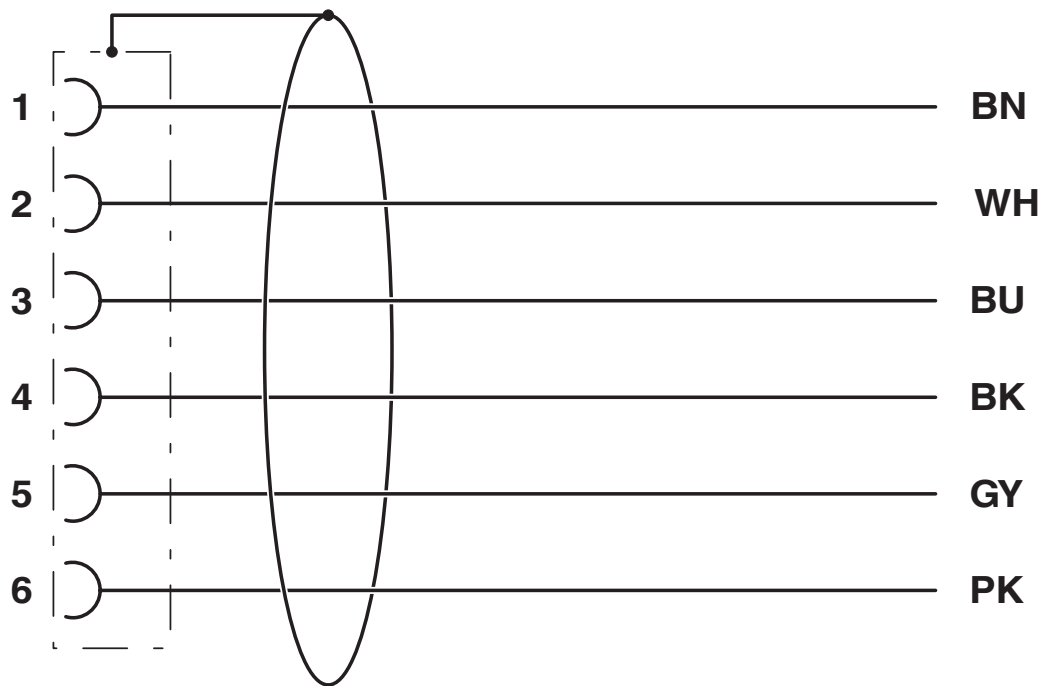
Schaltplan
