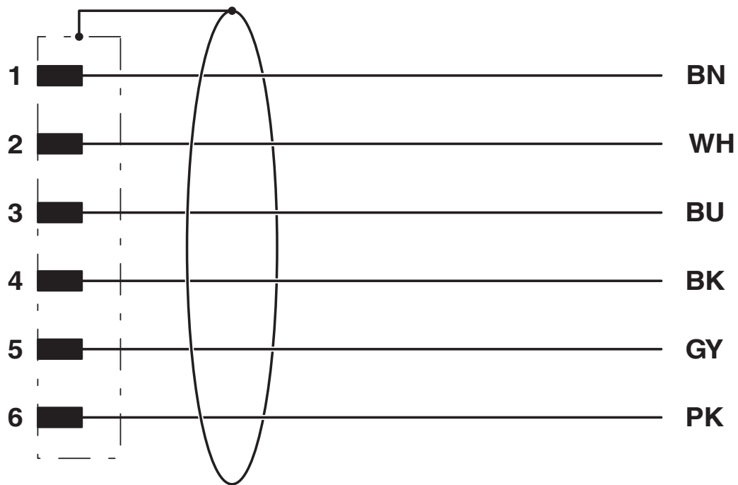
Kontaktbelegung des M8-Steckers
