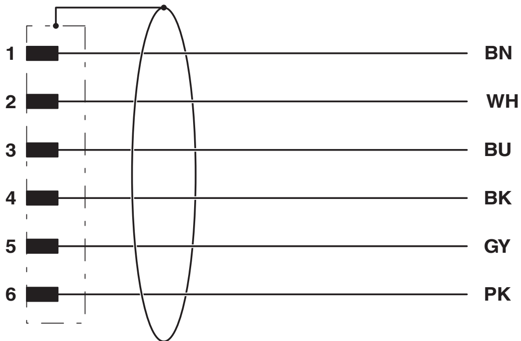
Schaltplan
