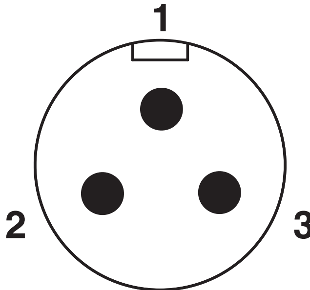
Schemazeichnung
