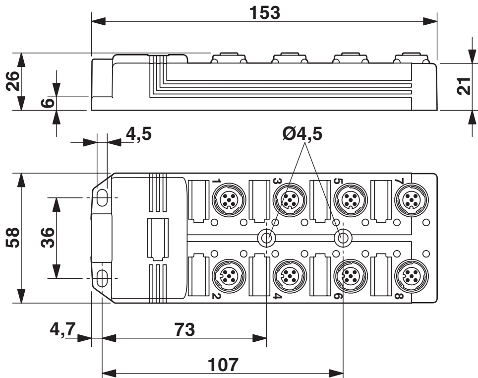
Maßzeichnung
