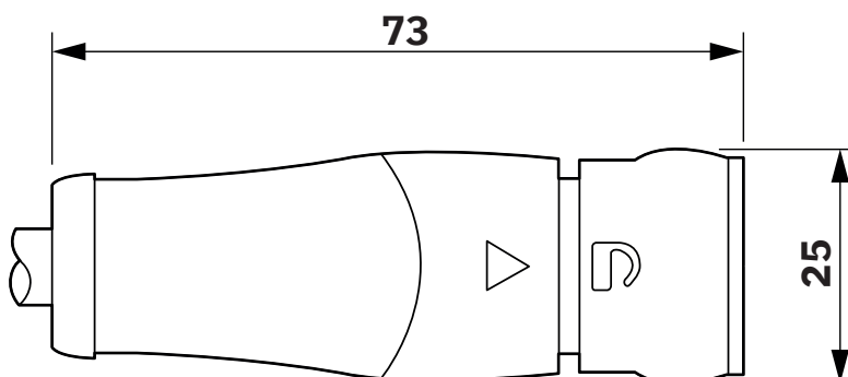
Maßzeichnung
