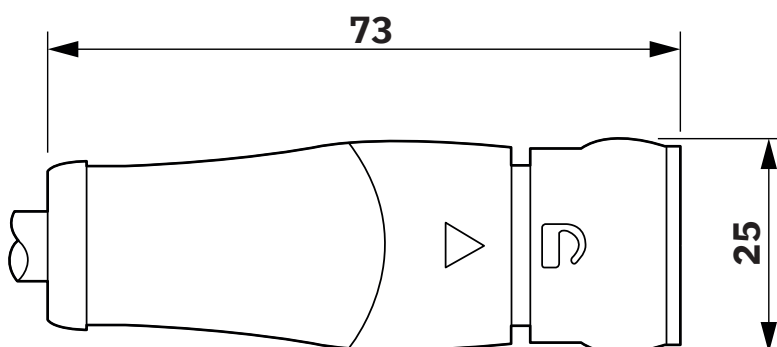
Maßzeichnung
