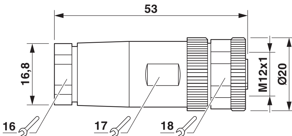
Maßzeichnung
