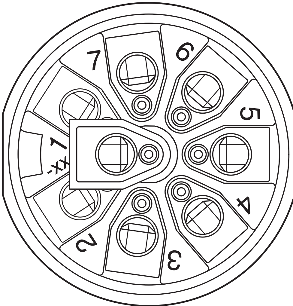
Schemazeichnung
