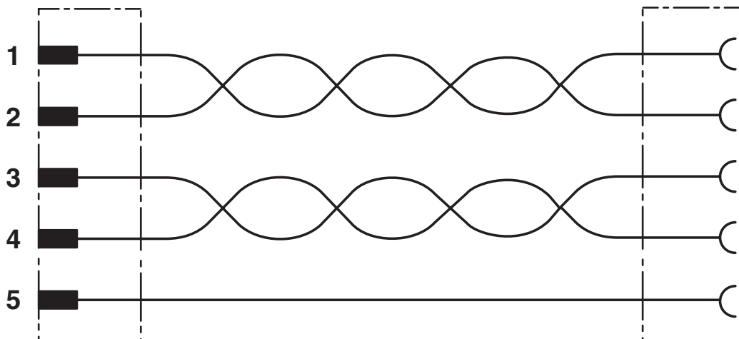
Schaltplan
