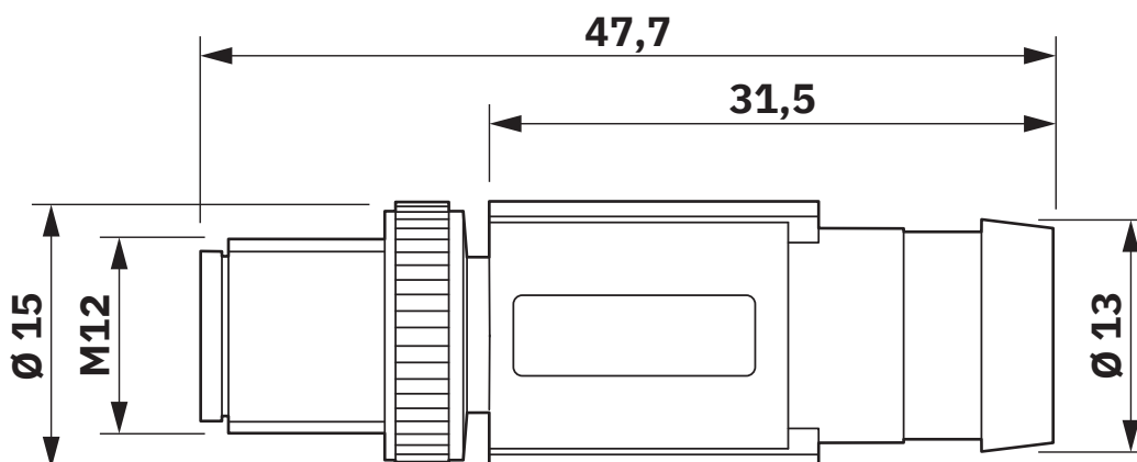
Maßzeichnung
